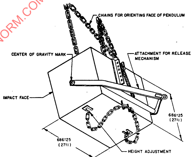
FIG. 9—PENDULUM
