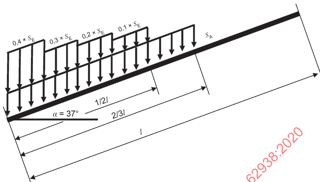
Figure 2 – Répartition de la charge sur l'éprouvette soumise à une inclination
