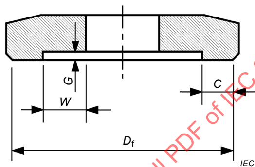
b) Flange design example b)
