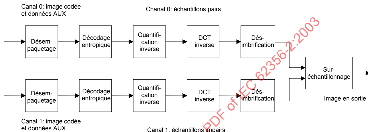
Figure 20 – Schéma-bloc du décodage
