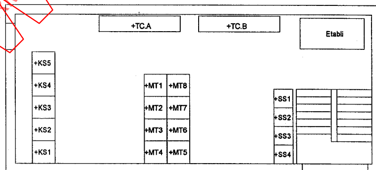
Figure 2d) – Dessin de base avec ajout de l'aménagement des armoires d'appareillage et de télécommunications
