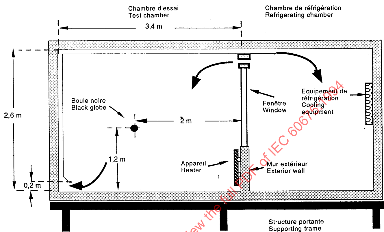
Figure A.1 — Exemple d'enceinte climatique Example of a climatic room
