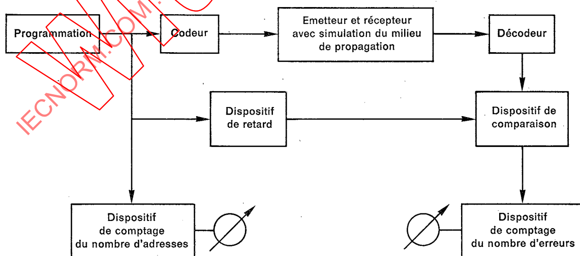
FIG. 6. — Exemple de montage de mesure.
