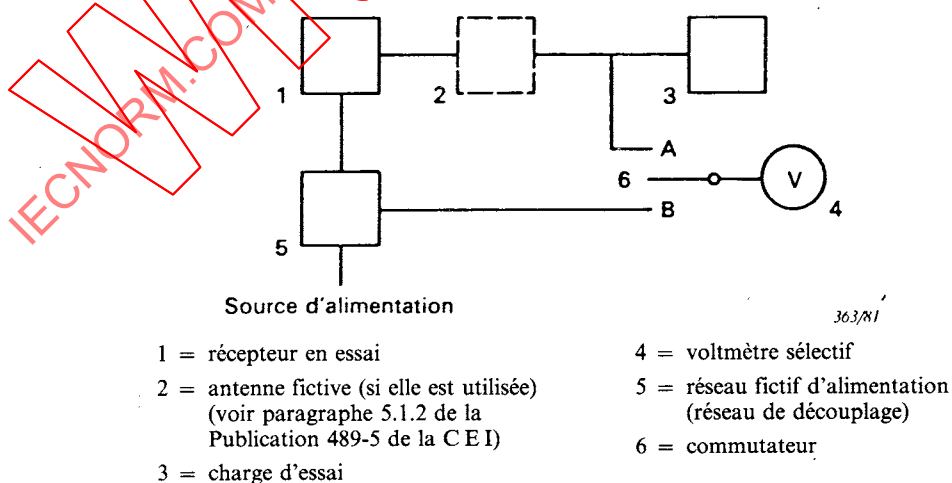
FIG. 7. — Montage de mesure des perturbations radioélectriques conduites aux bornes d'antenne et aux accès d'alimentation en courant alternatif.
