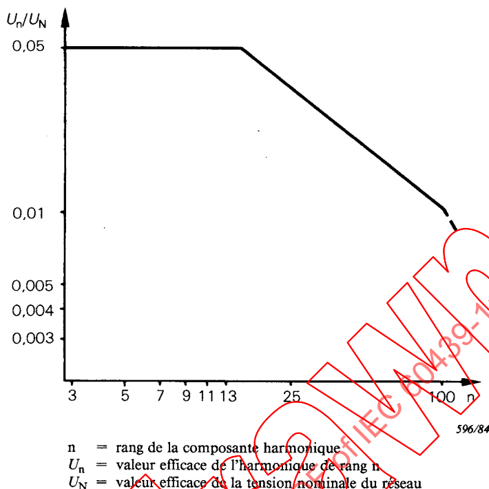
FIG. 2. — Composante harmonique maximale autorisée de la tension nominale du réseau.
