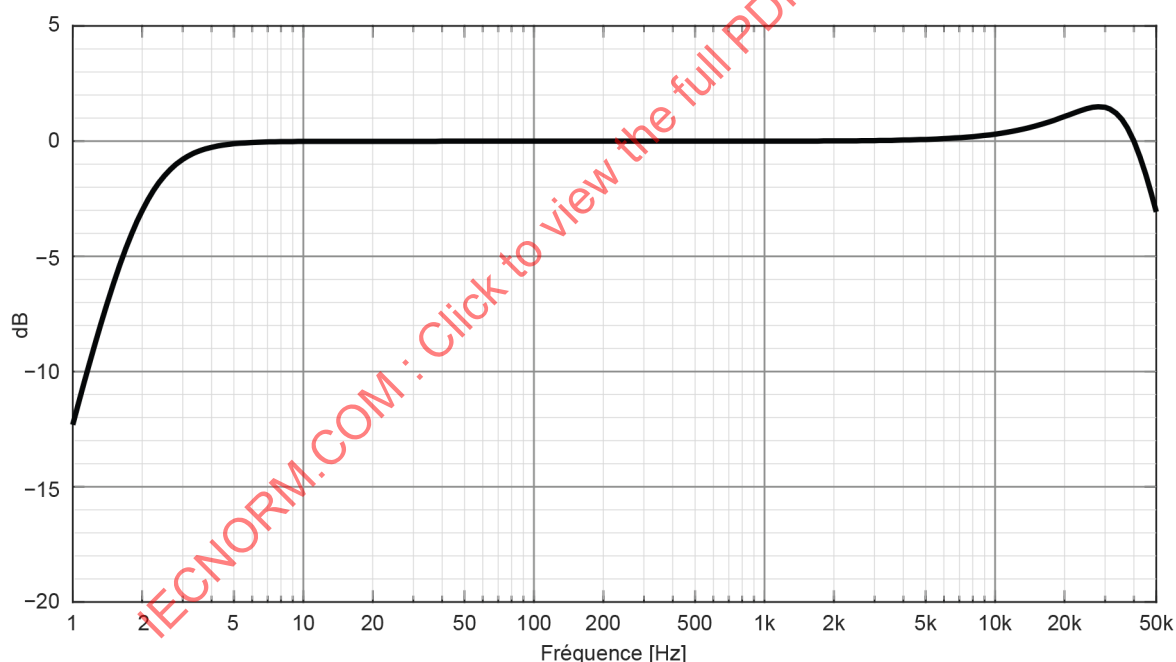
Figure A.1 – Exemple de courbe d'étalonnage d'un microphone représentant la réponse relative en dB en fonction de la fréquence avec un format de 10 dB/décade
