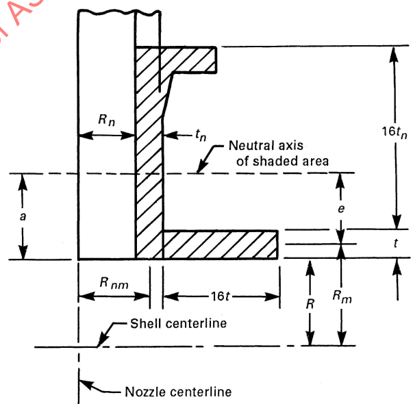
(d) Case B Nozzle With Integral Type Reinforcement
